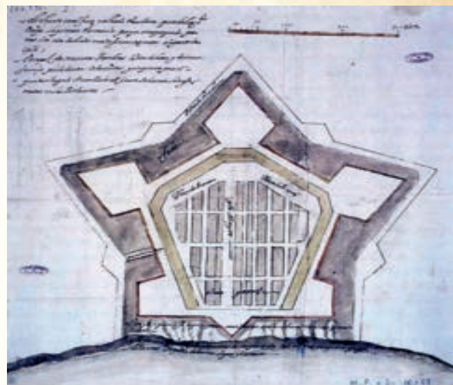
Planta del fuerte de La Mamora proyectado por Cristóbal de Rojas en 1614. A.G.S. Reproducción a partir del artículo de F.J. Bueno Soto (Aldaba) citado en nota 8.
